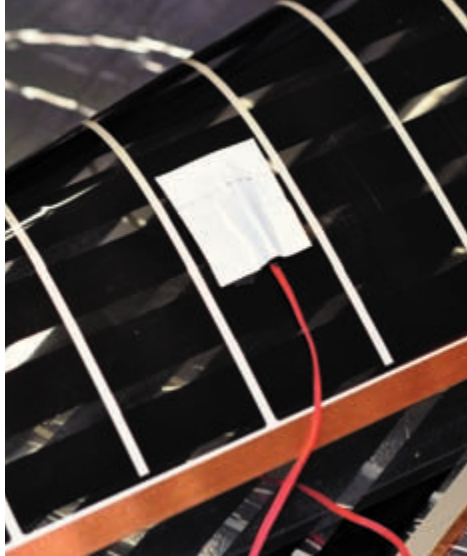
Рис. 25. Установленный и приклеенный датчик температуры пола. Вид снизу термопленки
