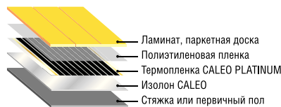
Рис. 28. Схема монтажа пленочного теплого пола под ламинат, паркетную доску
