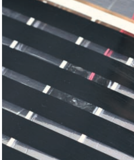
Рис. 26. Установленный и приклеенный датчик температуры пола. Вид сверху термопленки
