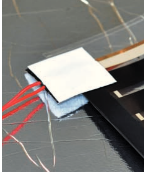
Рис. 20. Вид заизолированного контактного зажима с подключенными проводами
