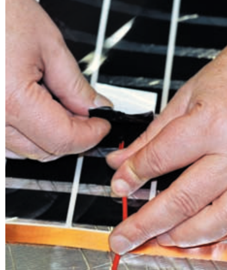
Рис. 24. Датчик прикрепляется к термопленке битумной изоляцией
