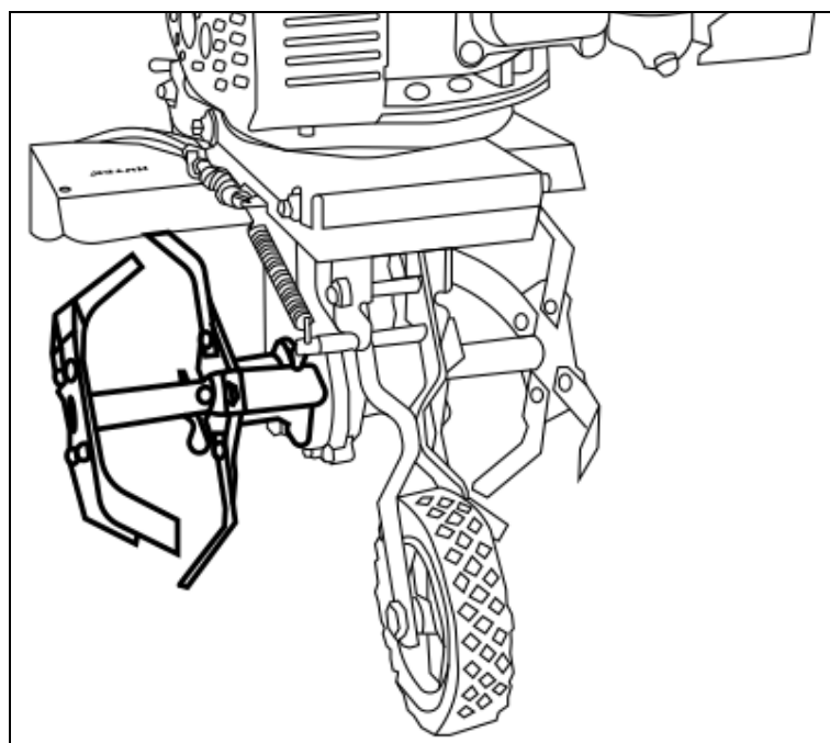
Рис. 7. Установка фрез
