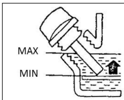
Рис. 11. Оптимальный уровень масла в картере
