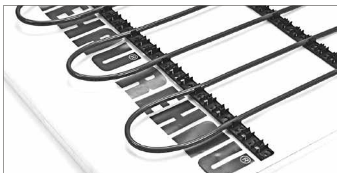
Рис. 21-19 Система RAUFIX
