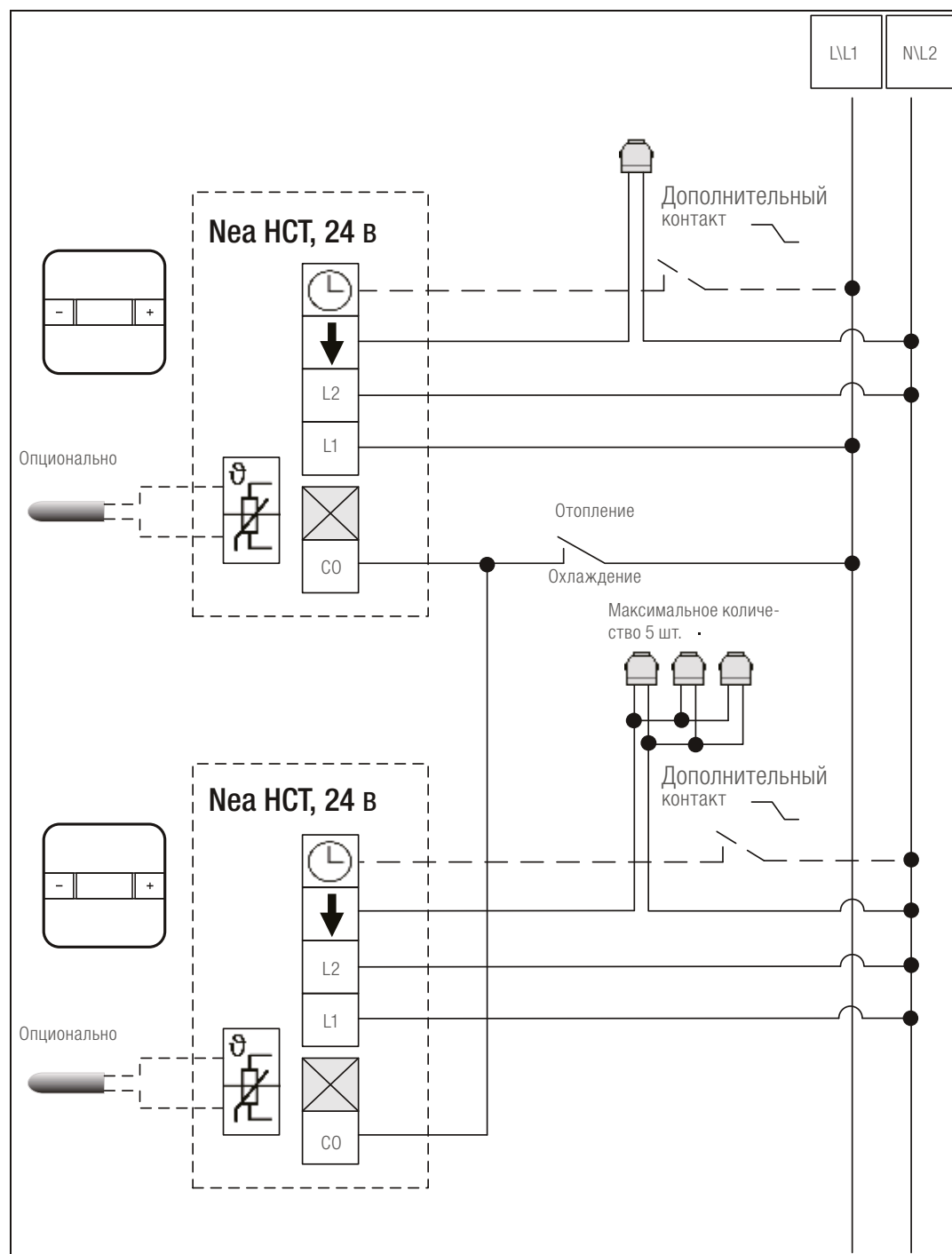
Рис. 26-10 Схема электрического подключения терморегуляторов Nea HCT без применения клеммной колодки Nea HC 24 В
