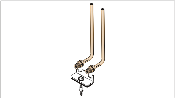
Рис. 13-5 Комплект Г-образных присоединительных трубок из меди
