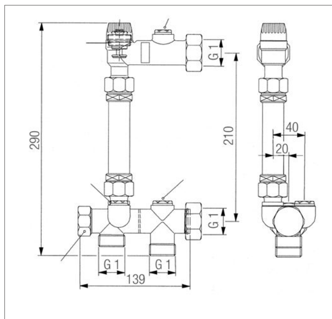
Рис. 17-14 Комплект установки теплосчетчика
