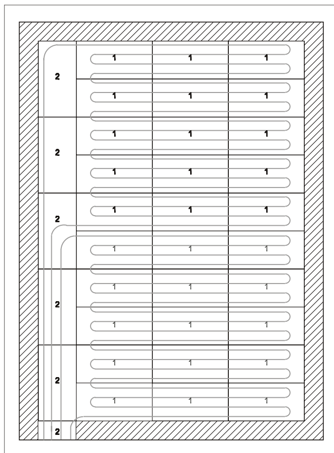
Рис. 22-7 Пример плана укладки труб в теплоизоляционные маты TS-14
