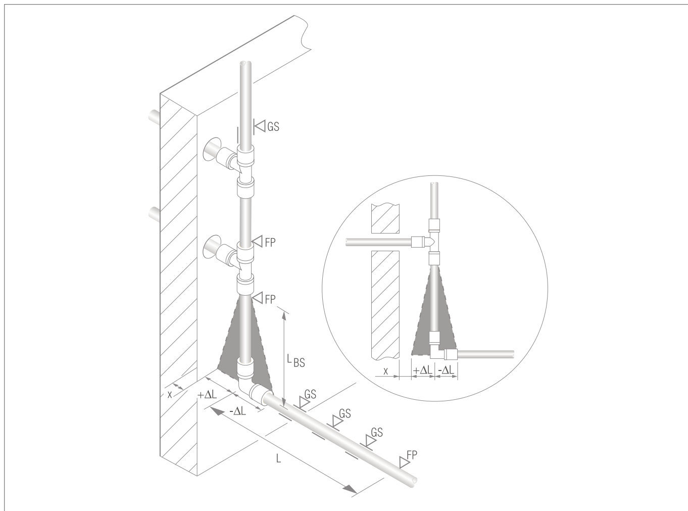
Рис. 8-1 Компенсатор
