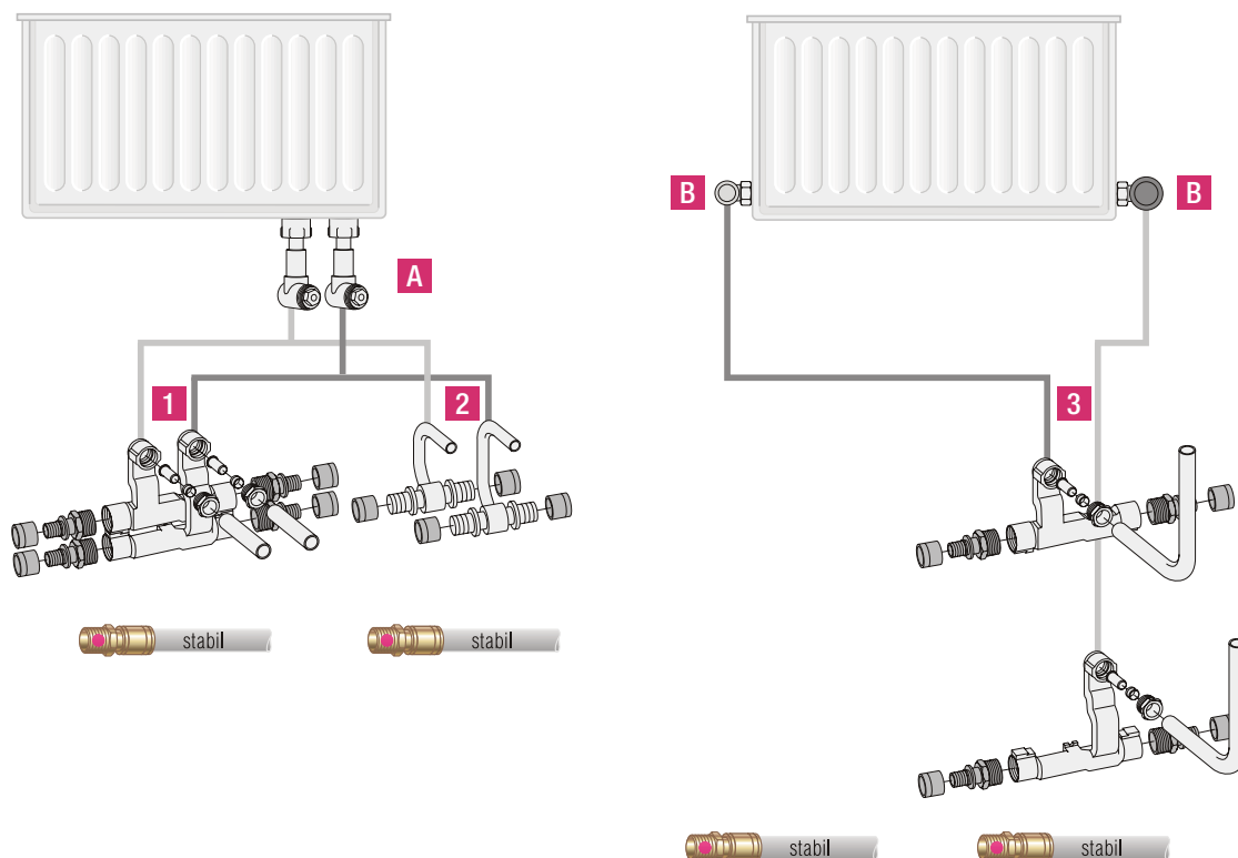
Рис. 16-3 Общий вид подключений к отопительным приборам в плинтусной разводке
