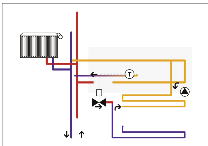
Рис. 25-6 Схема системы
