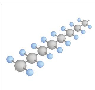
Рис. 1-3 Полиэтилен (PE)
