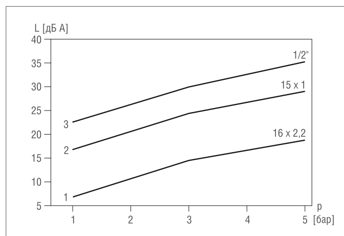
Рис. 6-3 Результат испытания Института им. Фраунхофера: сравнительный анализ шумоизолирующих характеристик материалов труб
