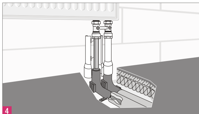
Рис. 13-10 Присоединение отопительного прибора с использованием присоединительного комплекта
