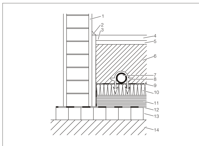
Рис. 21-41 Маты (комбинированная тепло-и шагозвукоизоляция) с гарпун-скобами для крепления отопительной трубы RAUTHERM S
