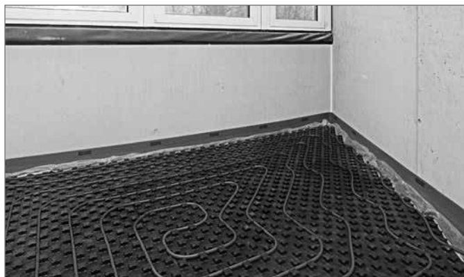
Рис. 21-22 Маты с фиксаторами Varionova с шагозвукоизоляцией 30-2 снизу
