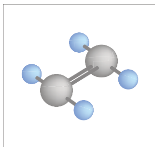
Рис. 1-1 Этилен
