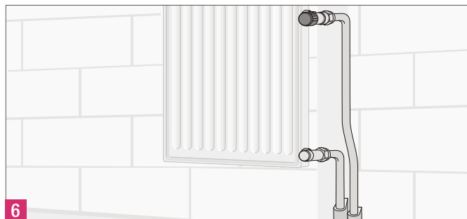
Рис. 14-12 Подключение к запорно-регулирующей арматуре радиатора с помощью переходника с наружной резьбой RAUTITAN MX
