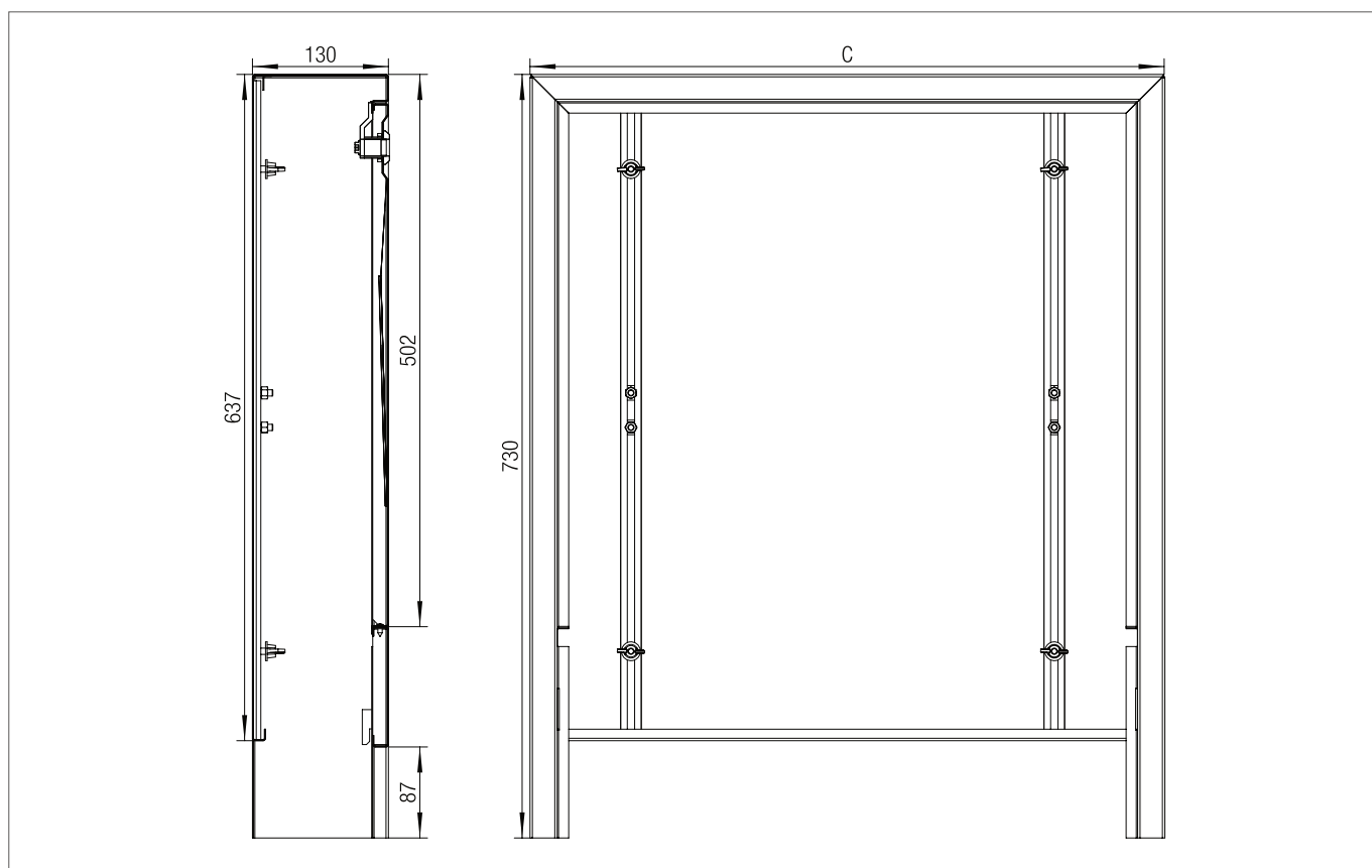
Рис. 24-10 Размеры распределительного шкафа AP
