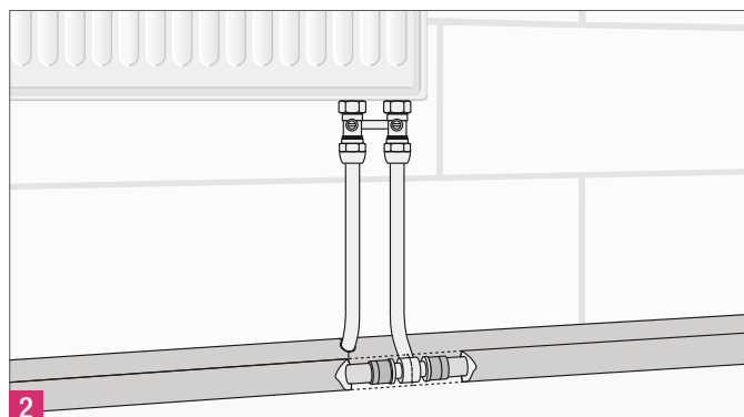
Рис. 13-6 Подключение отопительного прибора из пола при помощи Т-образных присоединительных трубок RAUTITAN
