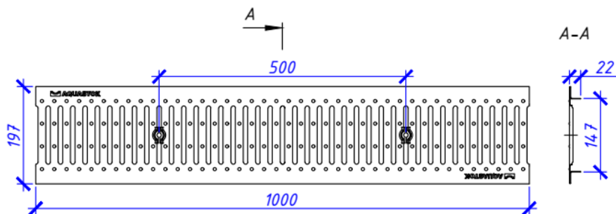
Решетка стальная щелевая оцинкованная DN150 A15
