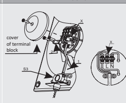
Pic.7 PARUS -02
