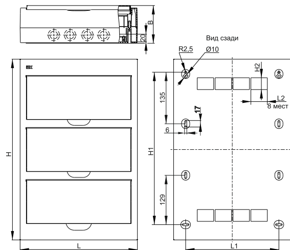
в) ЩРН-П-36 Продолжение рисунка 1
