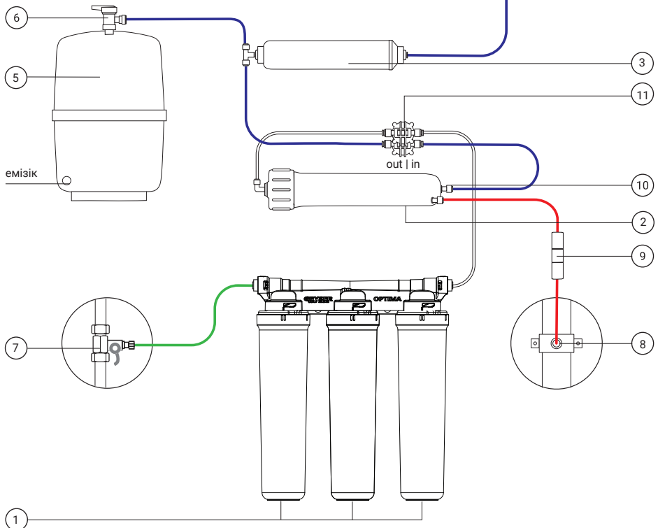
2-сур. Гейзер Престиж/Аллегро Оптиманы қосу схемасы
