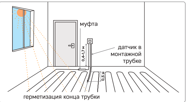
Рисунок 1. Монтаж терморегулятора и теплого пола
