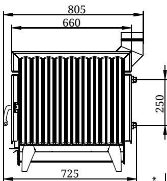
Рисунок 5. Габаритные размеры «Огонь-батарея 9Б» с выходом для трубы вверх
