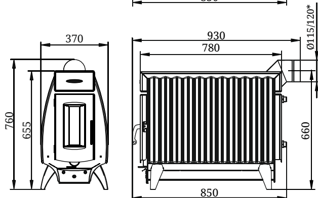
Рисунок 8. Габаритные размеры «Огонь-батарея 11Б» с выходом для трубы назад
