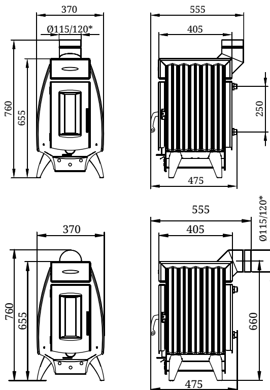
Рисунок 2. Габаритные размеры «Огонь-батарея 5Б» с выходом для трубы назад
