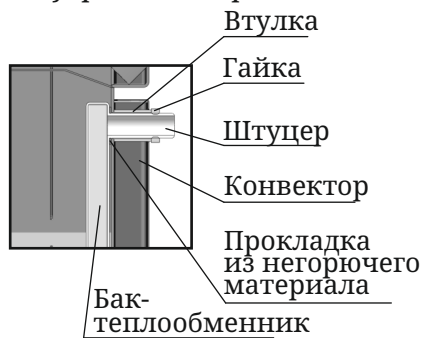
Рисунок 16. Демонтаж теплообменника
