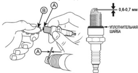
Рис. 21 Проверка зазора между электродами А – зазор В – шуп
