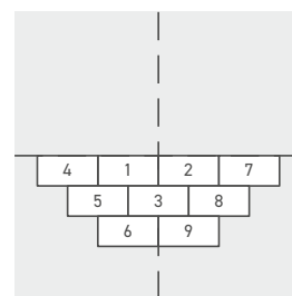
Укладка планок
