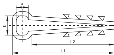
Рисунок 1 – Габаритные размеры хомута / Figure 1 – Overall dimensions of the clamp (5–10 ÷ 19–25 mm)
