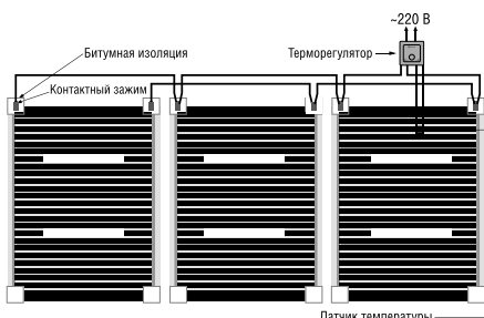
Датчик температуры
