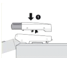
Монтаж демпфера
