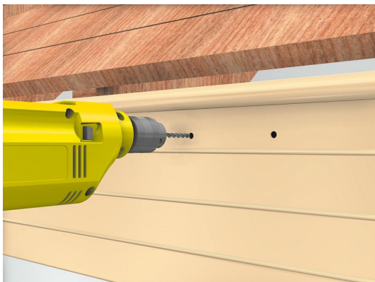
Рис. 27 Монтаж воронок PREMIUM и STANDARD на регулируемые крепления
