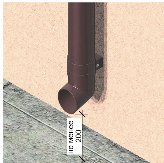
Рис. 44 Монтаж наконечника
