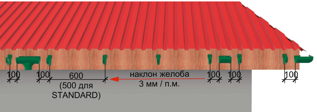
Рис. 8 Расположение кронштейнов
