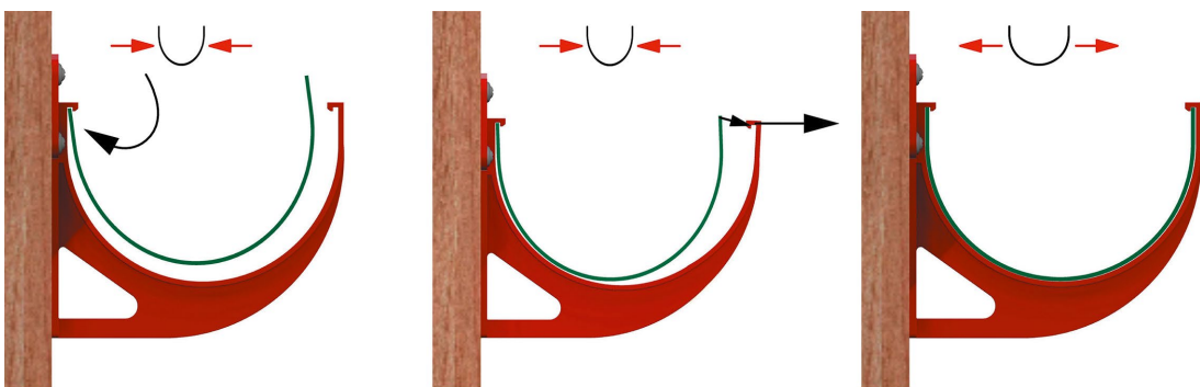
Рис. 21 Установка желобов в пластиковые кронштейны
