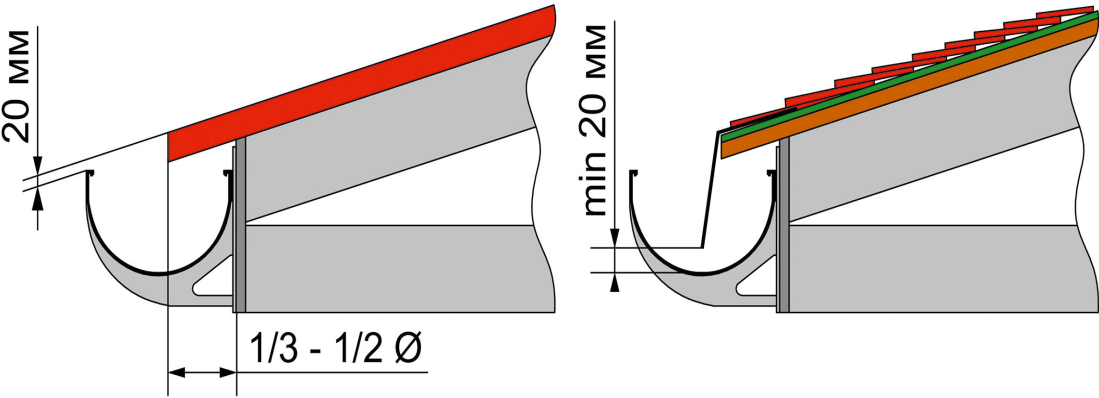
Рис. 5 Схема установки желоба водосточной системы Döcke
