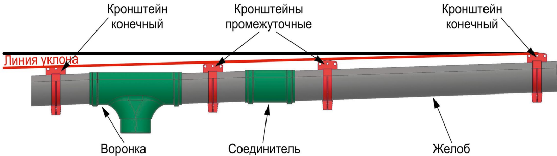
Рис. 6 Расположение водосбора относительно карниза
