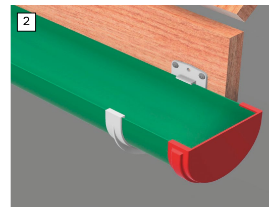
Рис. 31 Установка заглушки желоба
