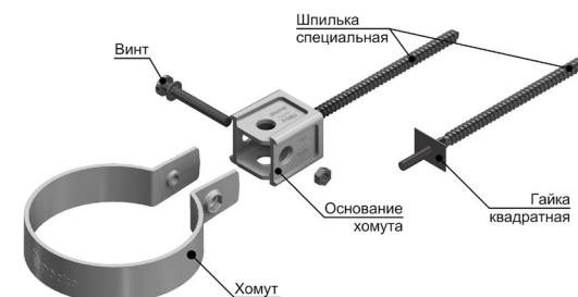
Рис. 35 Хомут PREMIUM универсальный и шпилька с гайкой
