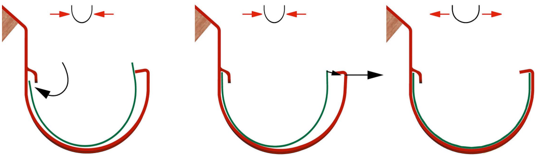
Рис. 22 Установка желобов в металлические кронштейны
