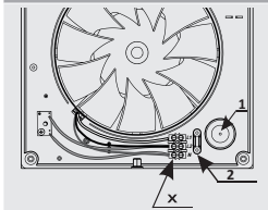
Рис. 2 AURA 6 / SILENT 6
