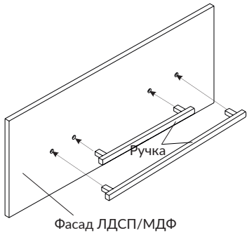
Схема установки ручки на фасад из ЛДСП/МДФ
