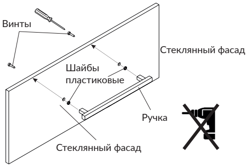
Схема установки ручки на стеклянный фасад
