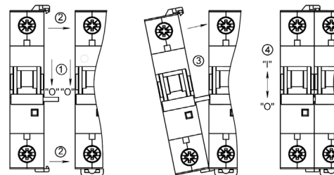
Рисунок Д.2 - Присоединение OptiDin HP, OptiDin PMMN к АВДТ OptiDin D63
