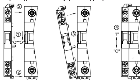
Рисунок Д.1 - Присоединение OptiDin MCK1, OptiDin MCK2, OptiDin MCKK2 к АВДТ OptiDin D63
