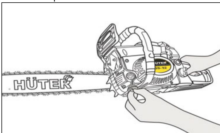
Рис. 13. Откручивание горловины масляного бака
