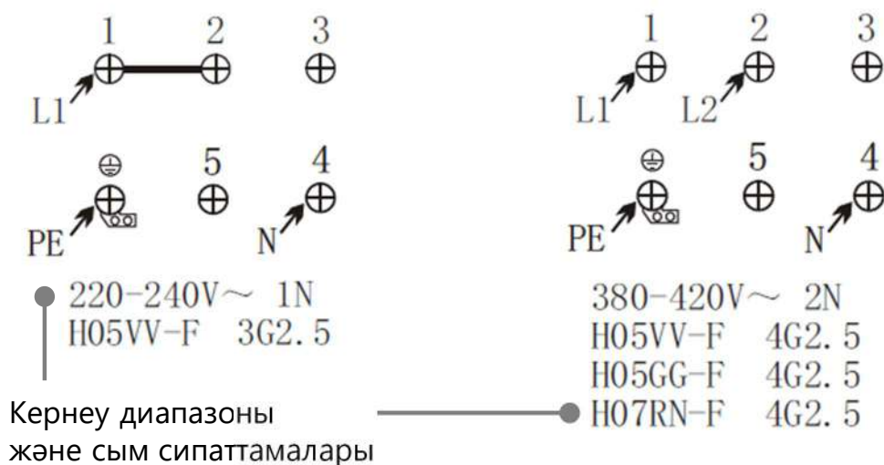
Электр қосылымының схемасы
