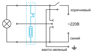
1. Светильник с подключением к сети ~220 В
