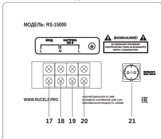
Рис. 5. Схема подключения 15000–30000ВА
