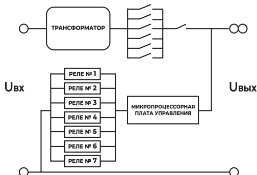
Рис. 6. Блок схема стабилизатора напряжения
