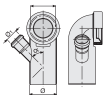
Отвод для унитаза белый с правым патрубком
