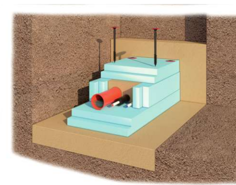
Тоннель тепло сберегающий в открытом грунте - XBS/ГВС/КНС
