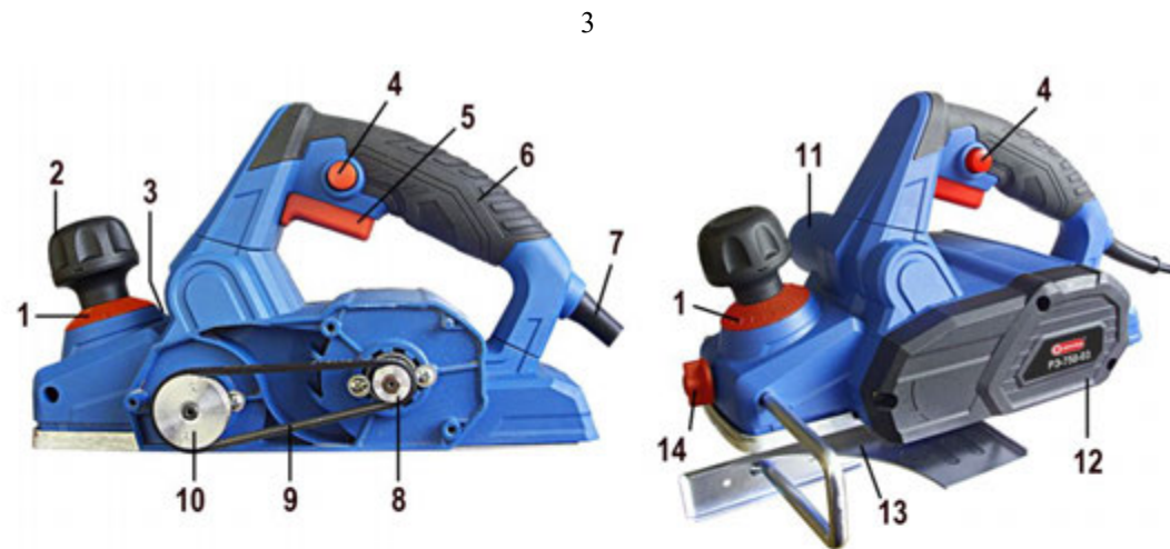
Внешний вид рубанка
