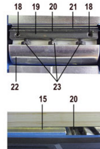
Установка ножей в рабочее положение
