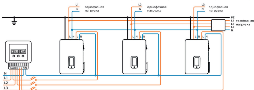
Рисунок 6. Подключение группы стабилизаторов напряжения к трехфазной пятипроводной сети при наличии однофазных и трехфазных нагрузок
