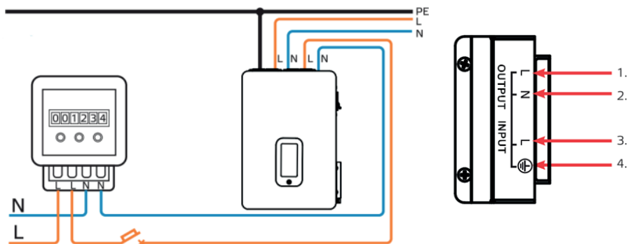
Рисунок 4. Подключение к однофазной сети
