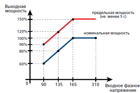
Рисунок 1. Зависимость выходной мощности от входного напряжения
