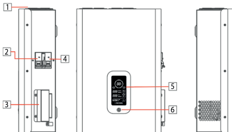
Рисунок 2. Внешний вид стабилизатора
