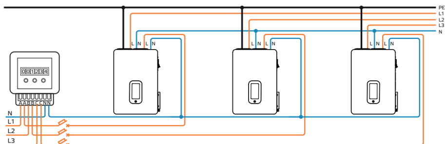
Рисунок 5. Подключение комплекта стабилизаторов напряжения к трех-фазной пятипроводной сети
